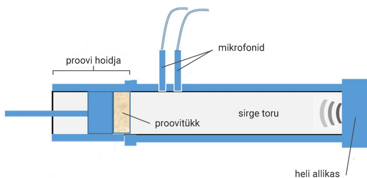
Joonis. 13. Impedantstoru joonis (Urdepilleta jt, 2022).
